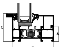
przekrój przez okno stałe
